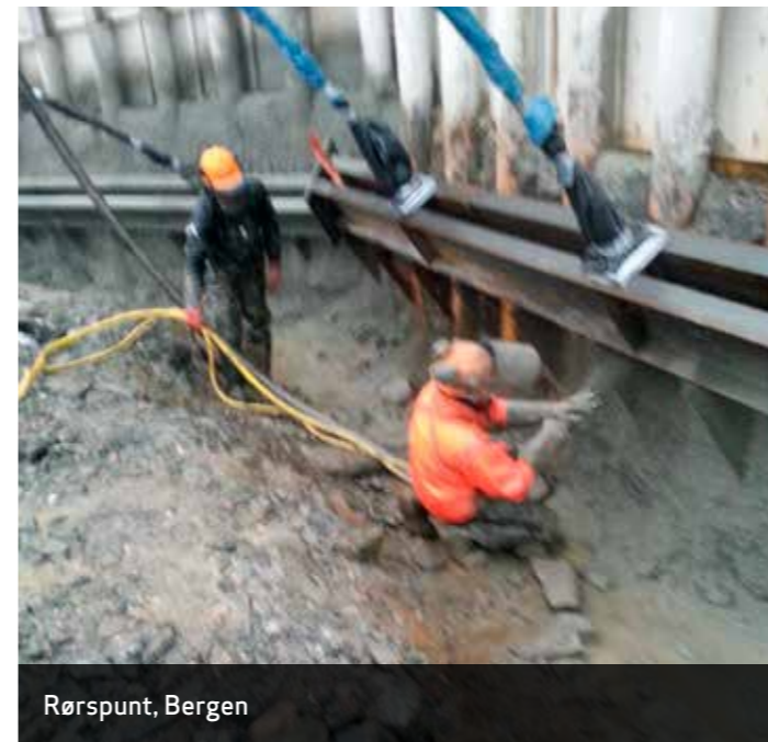
Rørspunt Haraldsplass, Bergen
